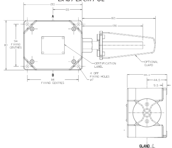
Ex ia / Ex em / UL
